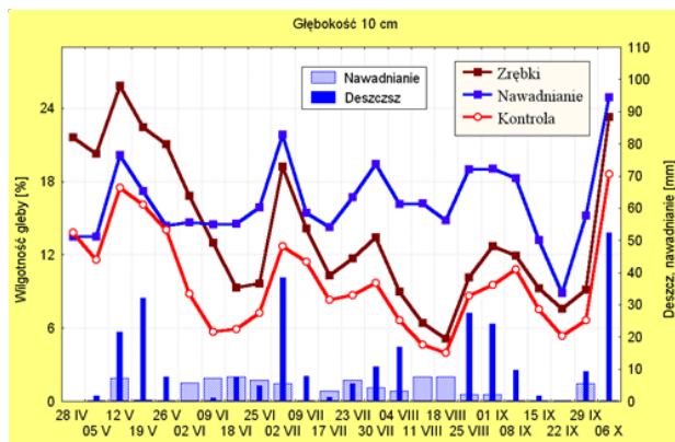
Rys. 6. Przebieg wilgotności gleby na głębokości 10 cm w sadzie przy różnych sposobach utrzymania gleby (W. Tredler)
