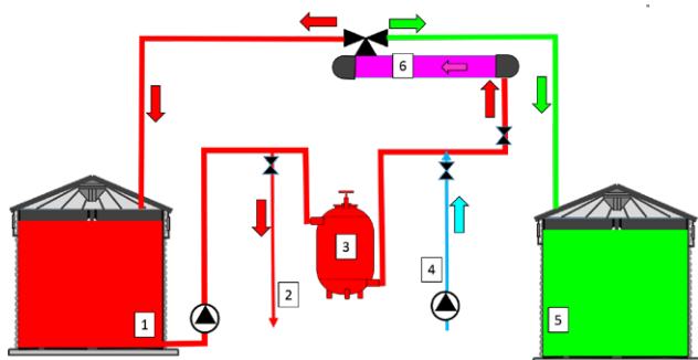
Rys. 15. Schemat systemu dezynfekcji wody za pomocą lampy UV-C. 1- zbiornik wody przed dezynfekcją, 2 - zrzut nadmiaru wody zanieczyszczonej, 3 - filtr piaskowy, 4- zasilanie wodą czystą, 5 - zbiornik na wodę po dezynfekcji, 6 lampa UV-C. (W. Treder)
