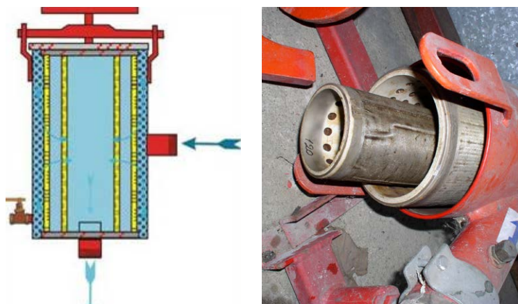
Fot. 25. Filtr z podwójnym wkładem siatkowym. (W. Treder)
