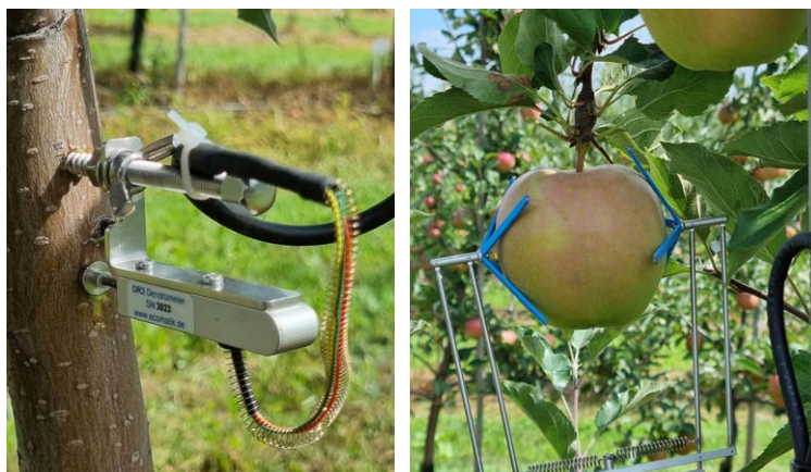
Fot. 75. Czujniki mikromorfometryczne do monitorowania mikrozmiian średnic pni i owoców (W. Tredler)
