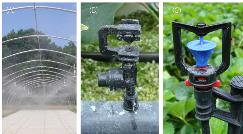
Fot. 51. Minizraszacze: umieszczają się wysoko na przewodach nad roślinami (A), na stopkach bezpośrednio nad łanem roślin (B), pod roślinami (C). (W. Treder)
