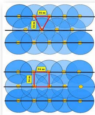
Rys. 22. Przykład rozstawienia zraszaczy w trójkąt lub kwadrat. Instalacja stała w sadzie o rozstawie 4 x 2,4 m (W. Treder)
