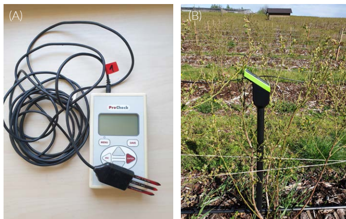
Fot. 71. Miernik wilgotności gleby z sondą pojemnościową (A) oraz bezprzewodowa sonda pojemnościowa (B) (W. Treder)
