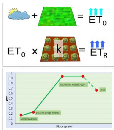
Rys. 29. Schemat metodyki wyznaczania potrzeb wodnych roślin (W. Treder)
