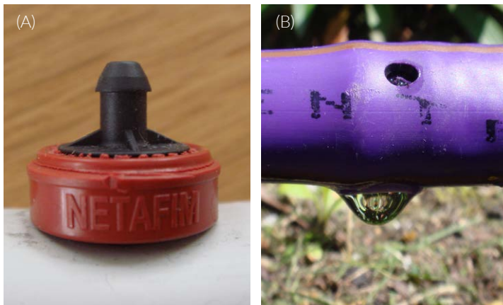
Fot. 56. Emiter kropłowy zamontowany na przewodzie polietylenowym (A) i linia kroplująca (B) (W. Treder)
