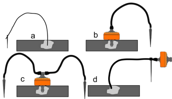
Rys. 27. Różne rodzaje emiterów kroplowych: kapilara (A), guzikowy ze stopką (B), guzikowy z rozdzielaczem (C) oraz zestaw kroplujący (D) (W. Treder)
